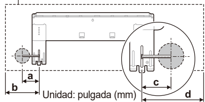
Estructura de la unidad interior
