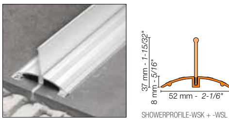
SHOWERPROFILE-WSK + -WSL
