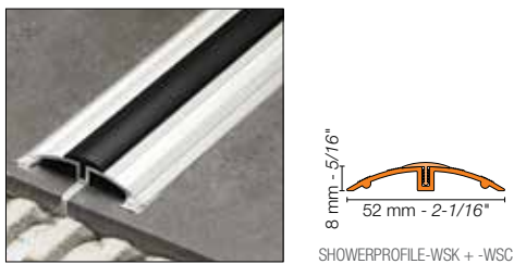
SHOWERPROFILE-WSK + -WSC
