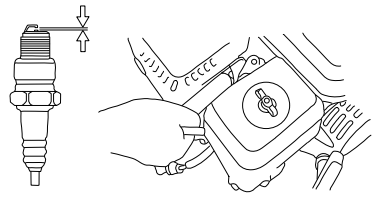
Figure 4-10. Bougie d'allumage
