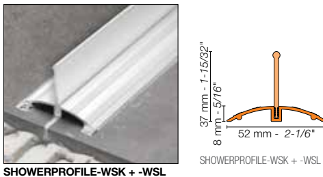
SHOWERPROFILE-WSK + -WSL
