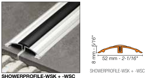
SHOWERPROFILE-WSK + -WSC
